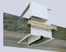
CORTAFUEGO EN FORJADO
