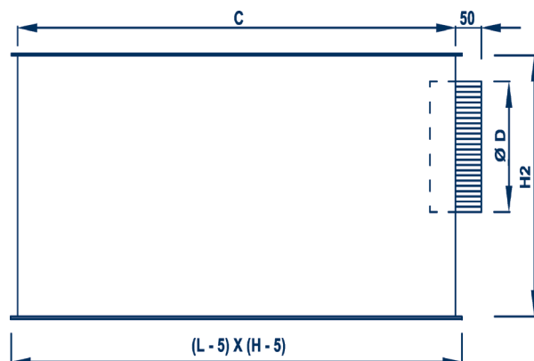
DHFP + PL/H (plenum horizontal)
